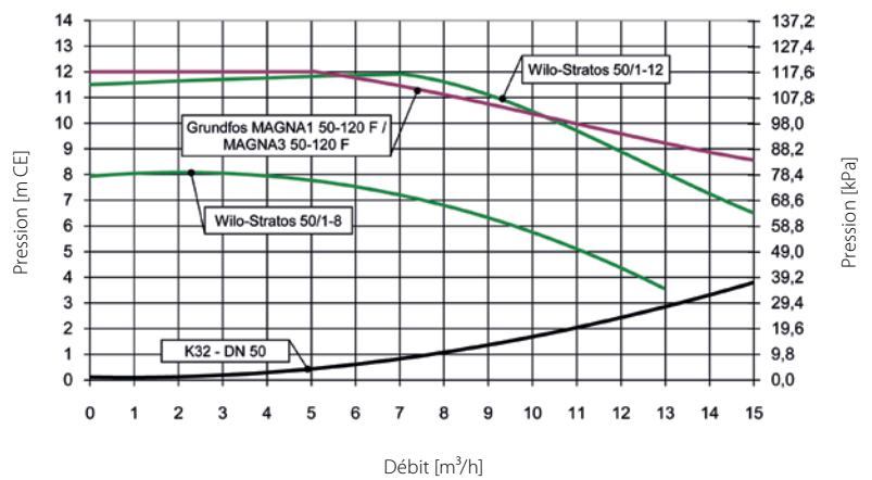
Diagramme de perte de charge HeatBloC K32
